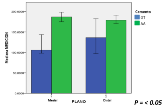
Figura 7. Comparación de microfiltración en micras de la superficie mesial y distal de los dos agentes cementantes.
