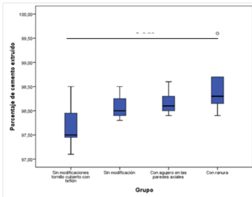
Figura 1. Comparación del porcentaje de cemento extruido en diferentes diseños de pilares para coronas implantoportadas
