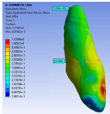
Imagen 10: Modelamiento del esfuerzo producido por el Gummetal en condiciones adecuadas.
