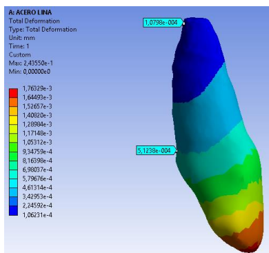
Imagen 9: Modelamiento de la deformación producida por el acero inoxidable en condiciones adecuadas.
