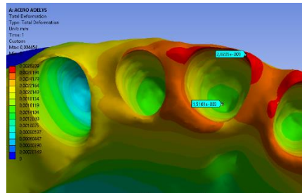
Imagen 4: Modelamiento de la deformación producida por el acero inoxidable en hueso disminuido
