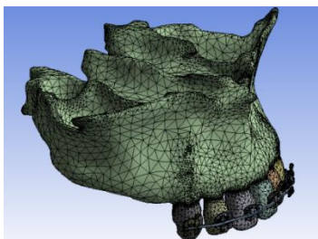
Imagen 1: Modelamiento de la unidad dentoalveolar.
