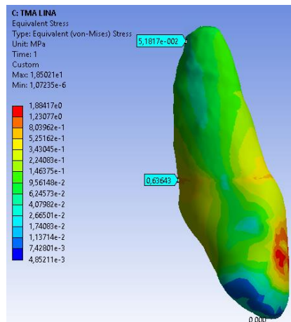
Imagen 10: Modelamiento del esfuerzo producido por el Gummetal en condiciones adecuadas.
