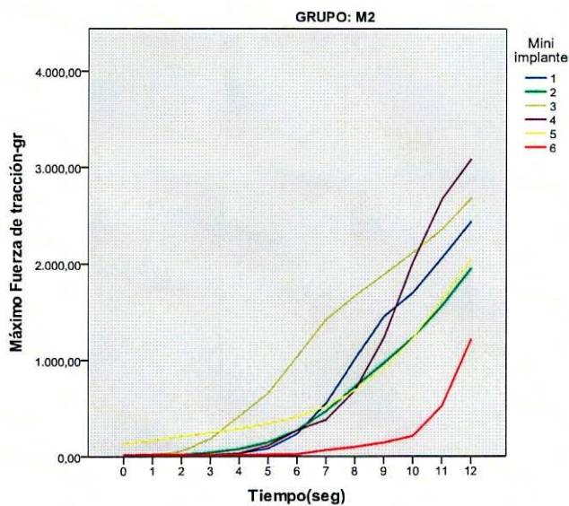
Figura 6. Relación Tiempo y fuerza de tracción ejercida en gr en cada mini implante – diseño nacional de mini implante (M2)
