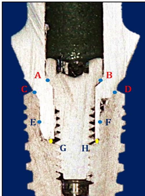
Fig. 4 Puntos de medición interfase Pilar/Implante
