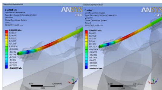
Figura 7a. Deformación evaluado sobre el arco de Gummetal.
