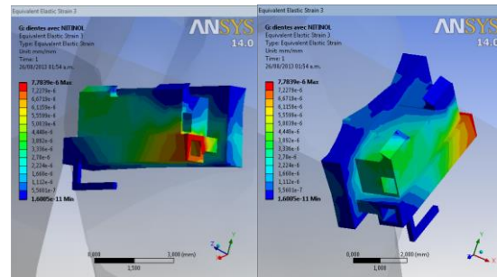
Figura 14a. Deformación evaluada en tubo molar con Gummetal. Figura 14b. Deformación evaluada en tubo molar con Nitinol
