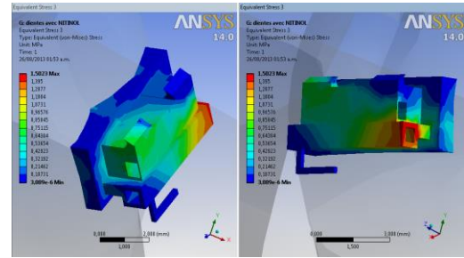
Figura 13. Esfuerzo evaluado en tubo molar con Nitinol
