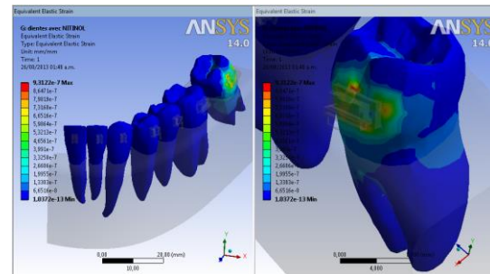
Figura 9. Esfuerzo evaluado sobre el diente con Nitinol
