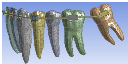
Figura. 1 Modelo de geometría inicial
