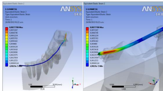
Figura 5. Esfuerzo evaluado sobre el arco de Gummetal
