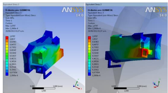
Figura 12. Esfuerzo evaluado en tubo molar con Gummetal
