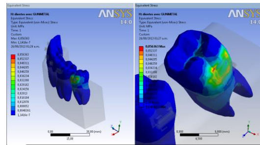
Figura 8. Esfuerzo evaluado sobre el diente con Gummetal
