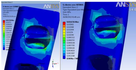
Figura 11a. Esfuerzo evaluado hueso alveolar con Gummetal. Figura 11b. Esfuerzo evaluado hueso alveolar con Nitinol
