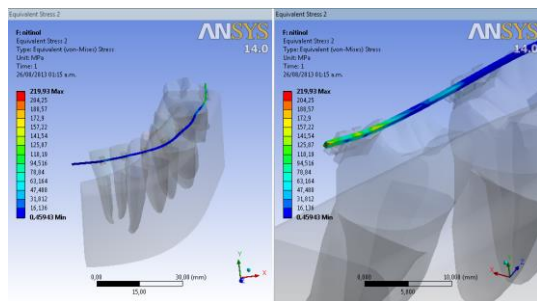
Figura 6. Esfuerzo evaluado sobre el arco de Nitinol
