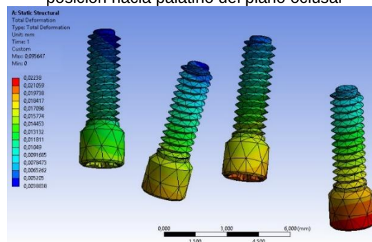
Figure 24 Deformaciones durante la aplicación de la carga en los tornillos protésicos en la prótesis metal-acrílica con implantes en posición hacia palatino del plano oclusal
