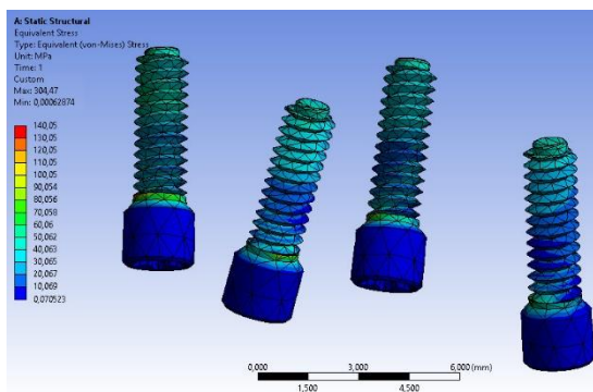
Figure 20 Esfuerzos durante la aplicación de la carga en los tornillos protésicos en la prótesis metal-acrílica con implantes en posición hacia palatino del plano oclusal
