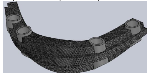
Figure 13 Barra 2 en titanio con implantes en posición del plano oclusal
