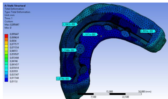
Figure 22 Deformaciones durante la aplicación de la carga vista del intaglio de la prótesis metal-acrílica con implantes en posición hacia palatino del plano oclusal
