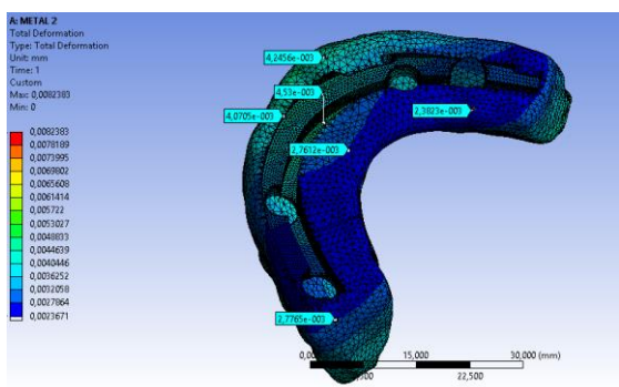
Figure 29 Deformaciones durante la aplicación de la carga vista del intaglio de la prótesis metal-acrítica con implantes en posición del plano oclusal
