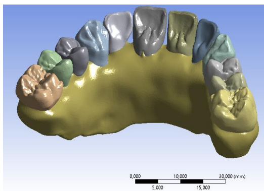
Figure 36 Prótesis total cerámica (barra en zirconio, dientes en disilicato) con implantes en posición del plano oclusal
