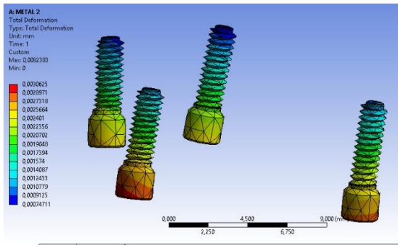
Figure 32 Deformación durante la aplicación de la carga en los tornillos protésicos de la prótesis metal-acrítica con implantes en posición del plano oclusal
