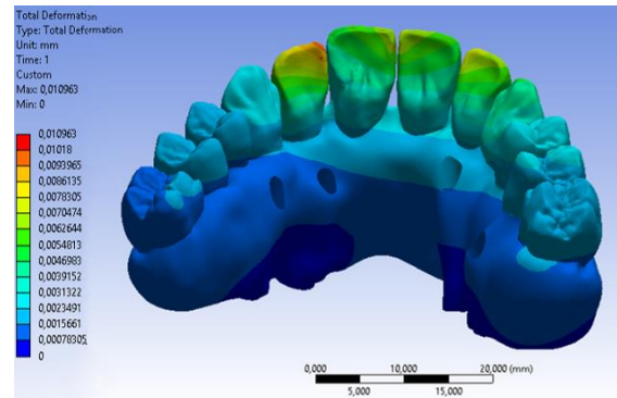
Figure 50 Deformaciones durante la aplicación de las cargas en la prótesis con la barra copy milled en zirconio con implantes en posición hacia palatino del plano oclusal y coronas en disilicato de litio
