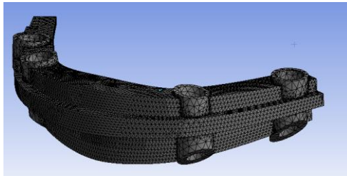
Figure 15 Enmallado de la barra
