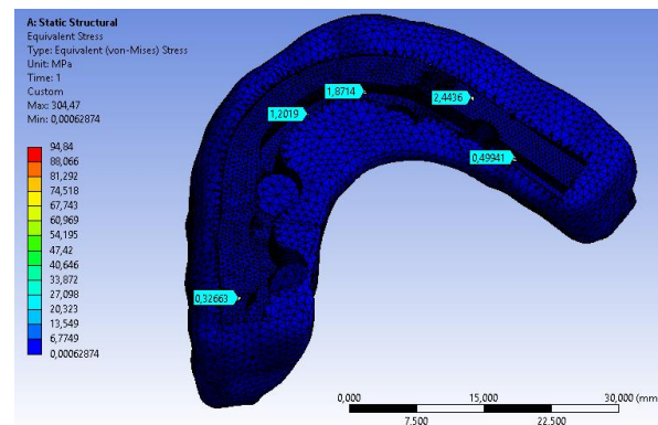
Figure 18 Esfuerzos durante la aplicación de la carga vista del intaglio de la prótesis metal-acrílica con implantes en posición hacia palatino del plano oclusal
