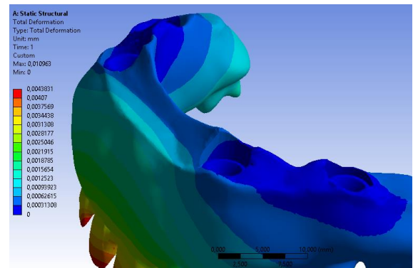
Figure 43 Deformaciones durante la aplicación de las cargas en la prótesis con la barra copy milled en zirconio con implantes en posición del plano oclusal y coronas en disilicato de litio vista del intaglio
