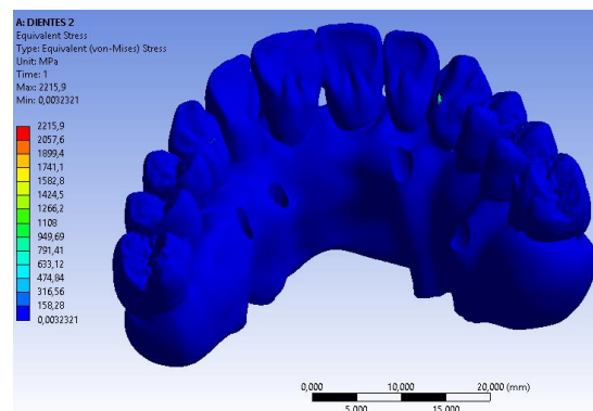
Figura 46 Esfuerzo durante la aplicación de las cargas en la barra copy milled en zirconio junto con las coronas en posición hacia palatino del plano oclusal. Se aprecia que el esfuerzo máximo se presentó donde la barra entra en contacto con los dientes en la zona cervical. El máximo valor en dicho punto fue de 200.18 MPa, incrementándose un 90% aproximadamente con respecto al modelo 3.
