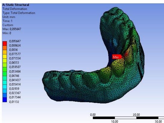
Figure 21 Deformaciones durante la aplicación de la carga vista oclusal de la prótesis metal-acrílica con implantes en posición hacia palatino del plano oclusal
