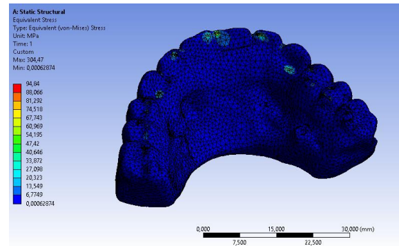
Figure 17 Esfuerzos durante la aplicación de la carga vista oclusal de la prótesis metal-acrílica con implantes en posición hacia palatino del plano oclusal
