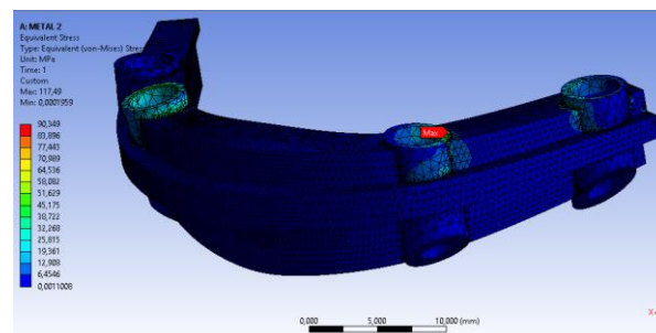
Figure 30 Esfuerzos durante la aplicación de la carga en la barra en titanio con implantes en posición del plano oclusal
