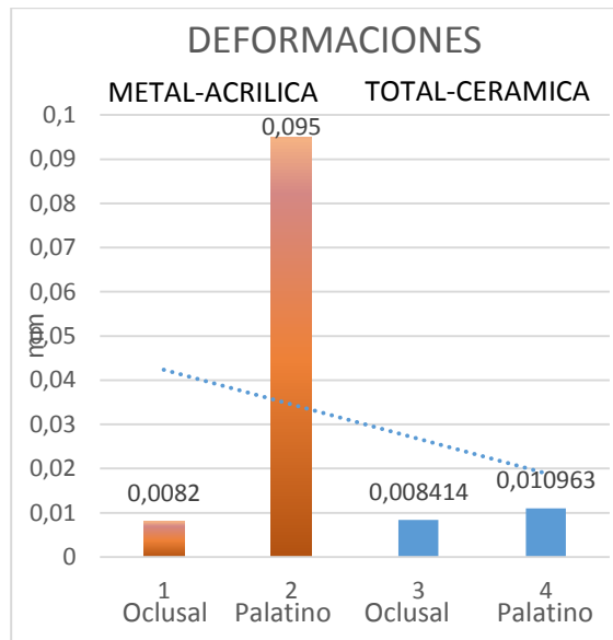
Grafica 2 Comparación de deformaciones en las prótesis híbridas metal acrílica y total cerámica
