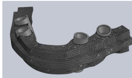
Figure 12 Barra 1 en titanio con implantes en posición hacia palatino del plano oclusal
