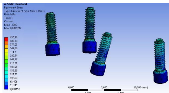
Figure 41 Esfuerzo durante la aplicación de las cargas en los tornillos protésicos de la barra copy milled en zirconio junto con las coronas en disilicato de litio con implantes en posición del plano oclusal
