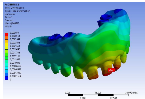
Figure 51 Deformación durante la aplicación de las cargas en barra de zirconio con implantes en posición hacia palatino del plano oclusal
