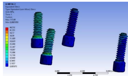
Figure 27 Esfuerzos durante la aplicación de la carga en los tornillos protésicos de la prótesis metal-acrílica con implantes en posición del plano oclusal
