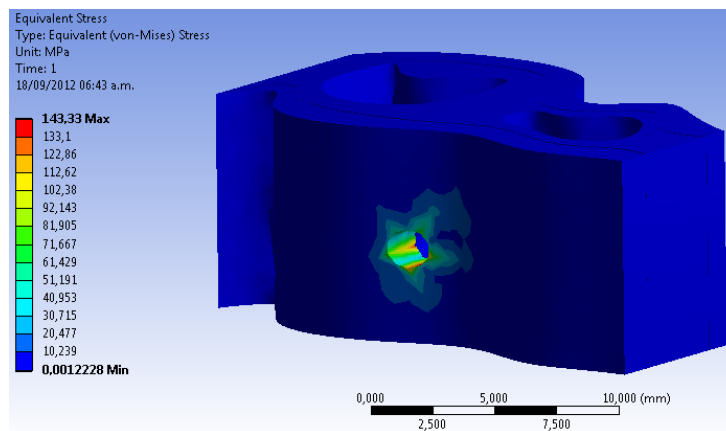
Fig. 4 Esfuerzo evaluado sobre el hueso con el nicho de 1.4 mm, relacionado con la técnica PressFit.
