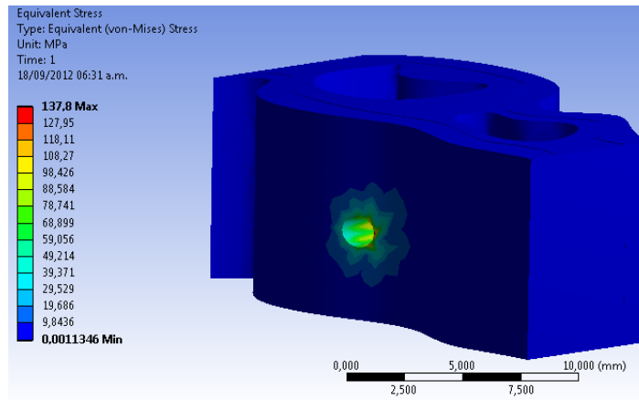
Fig.3 Esfuerzo evaluado sobre el hueso con nicho de 1.6 mm, relacionado con la técnica PressFit.
