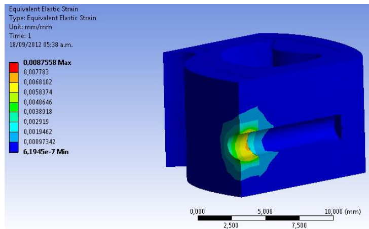
Fig. 2.1 Deformación del hueso con el nicho de 1.8 mm
