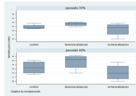
Gráfico 1. Tamaño de los poros por concentración de peróxido
